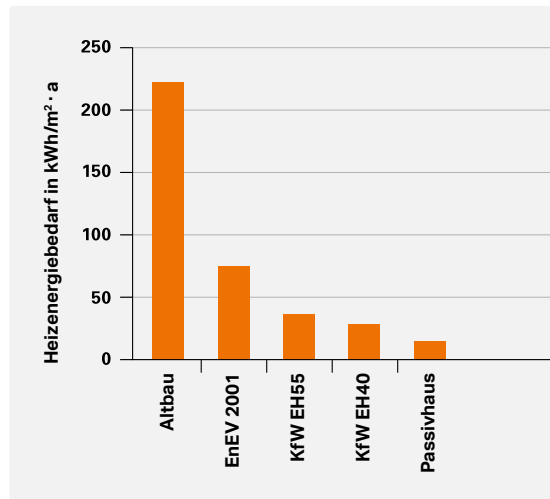
Dank der Innovationen hin zu modernen Ziegeln liegt der Heizenergiebedarf 1 der damit errichteten Häuser heute bei unter 30 kWh/(m 2 · a).
