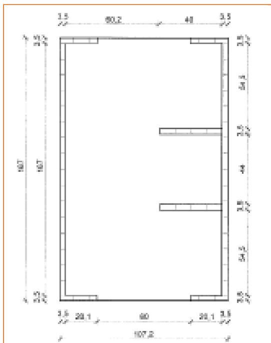
Bild 4: Grundriss des Reihenhauses [1]
